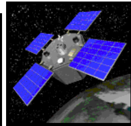
ACRIMSAT ACRIM3 (2000 -->)
